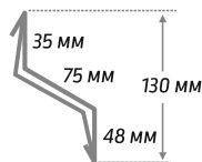
Подвійна ламель
