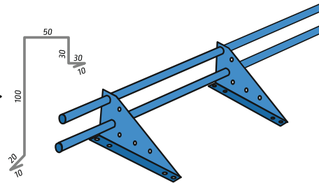
Трубчастий снігозатримувач
