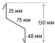
Одинарна ламель
